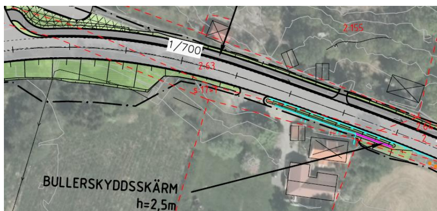
Förslag att förlänga befintlig bullerskyddsskärm öster om Tjuvkils vägskäl. Utsnitt ur vägplanens illustrationskarta.
