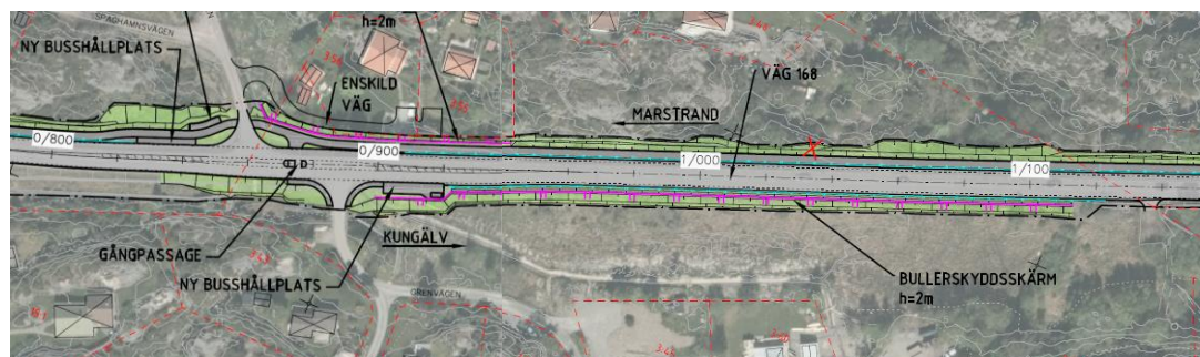
Föreslagen bullerskyddsskärm öster om Toftebergsvägens/Grenvägens anslutning till väg 168. Längd 214 m, höjd 2 m. Genomsiktlig skärm på vissa avsnitt. Utsnitt ur vägplanens illustrationskarta.
