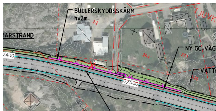
Föreslagen bullerskyddsskärm vid Spaghamsnvägen. Utsnitt ur vägplanens illustrationskarta.
