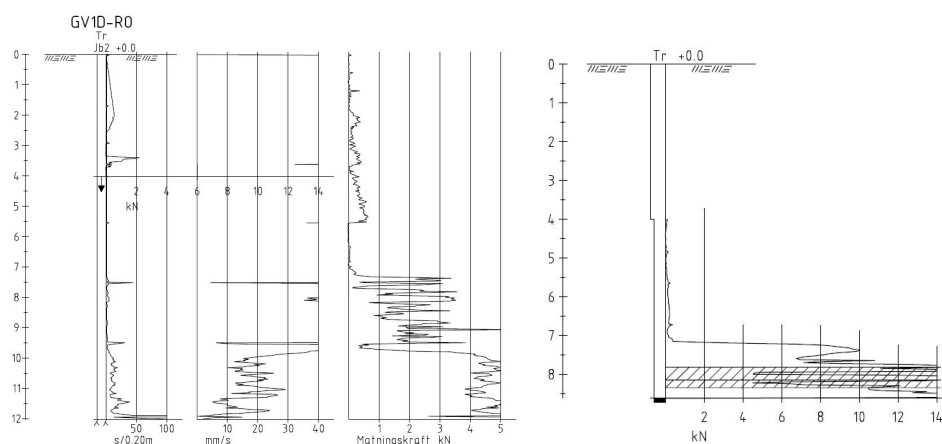
Figur 15. Utförda trycksondering och jord- bergs sondering i provtagningspunkt GV1d-Röd.
