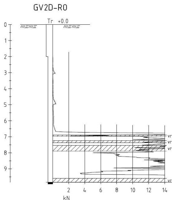
Figur 16. Utförda trycksonderingar i provtagningspunkterna GV2d-Röd
